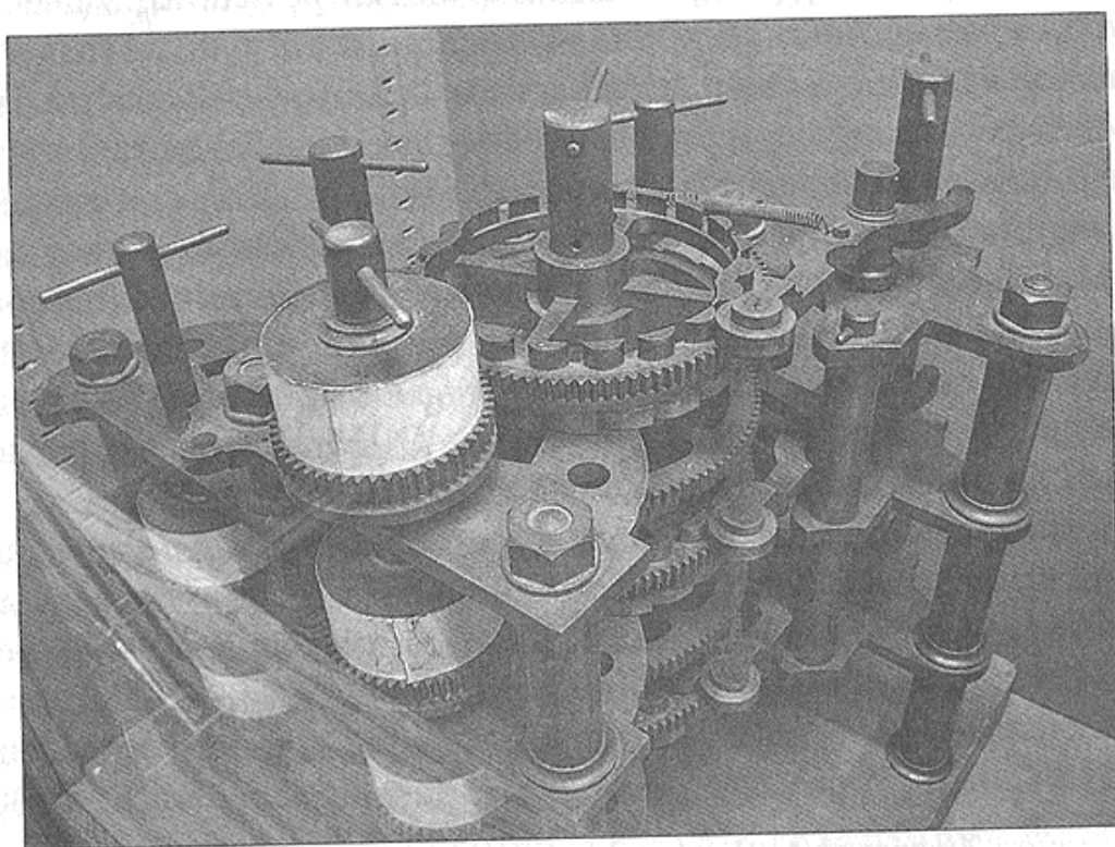
Рис. 3.1. Машина Бэббиджа
