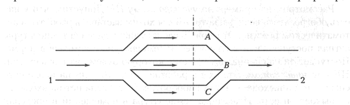
Рис. 3.9. Схема «трубопровода»
