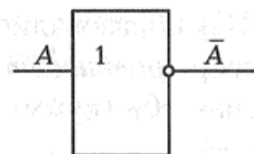
Рис. 3.10. Логическая схема НЕ
