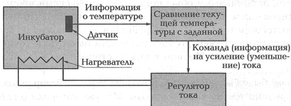
Рис. 2.3. Схема термостата
