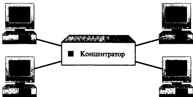
Рис. 9.2. Топология «звезда»
